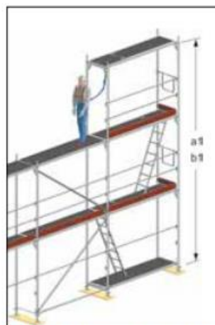
Bild 16: Fästning över huvudhöjd
