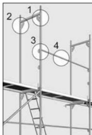
Bild 6: Översikt över fästpunkterna 1-4 (OBS! Fästpunkt 4 - EJ tillåtet på alu-SpeedyScaf).
